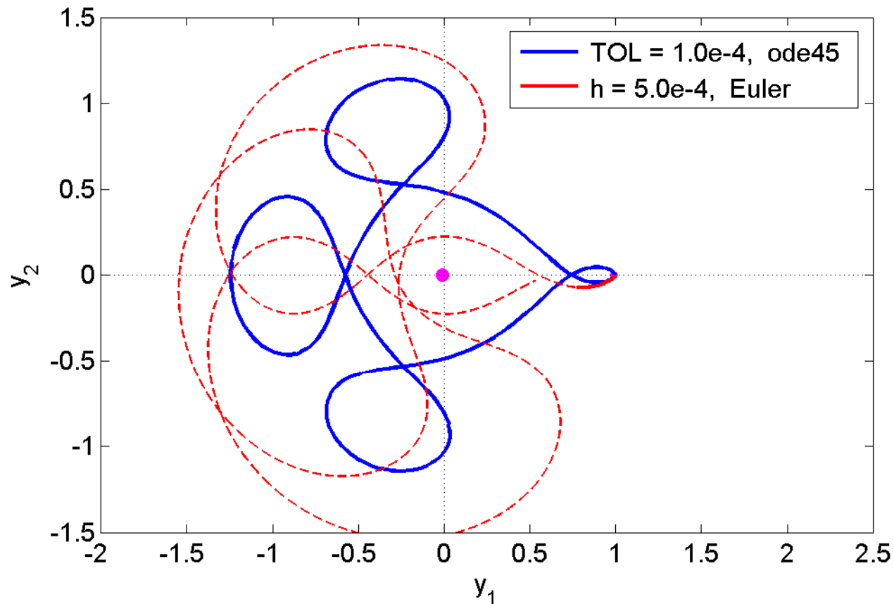
Arenstorf-Orbit
